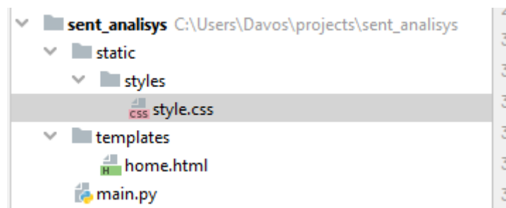
Рис. 3.47. Структура проєкту
