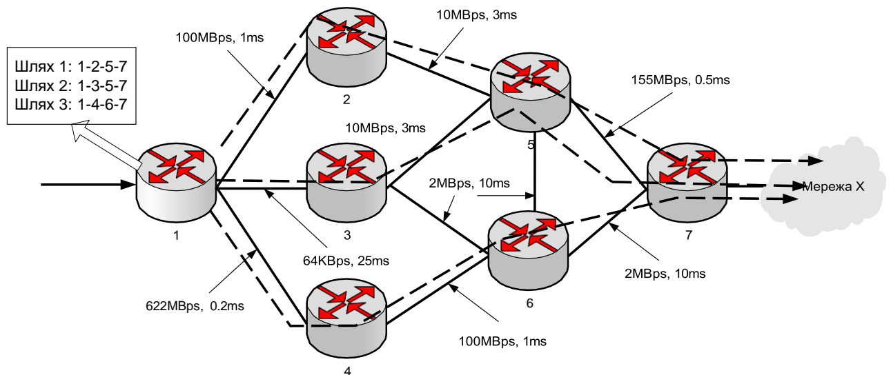
Рисунок 1.4 – Реалізація багатокільніною маршрутизації
