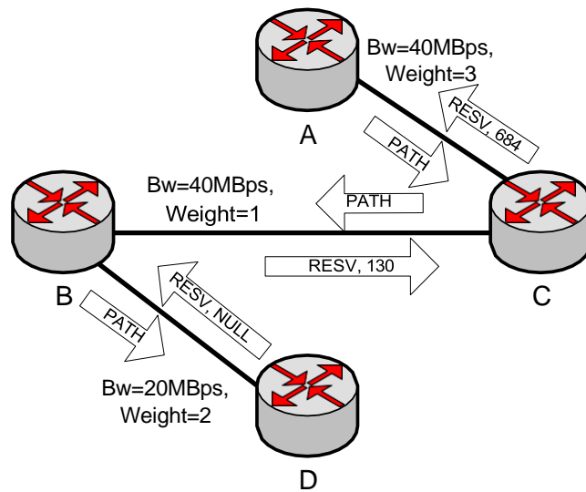
Рисунок 3.3 – Створення тунелю та резервування ресурсів протоколом RSVP-TE
