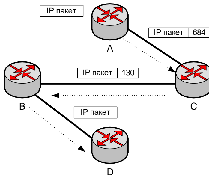
Рисунок 3.4 – Пересилання пакетів від вузла A до D через створений тунель
