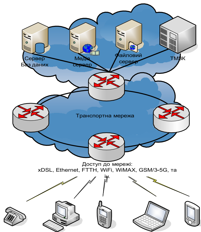
Рисунок 1.2 – Структура мереж наступного покоління
