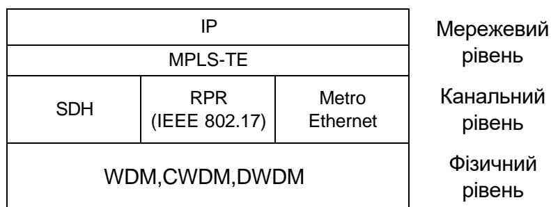
Рисунок 3.14 – Структура транспортних технологій
