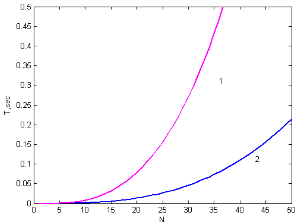
Рисунок 3.32 – Залежність часу розв'язання задачі від розмірності мережі 1- модель Галаггера, 2-евристичний алгоритм релашування
