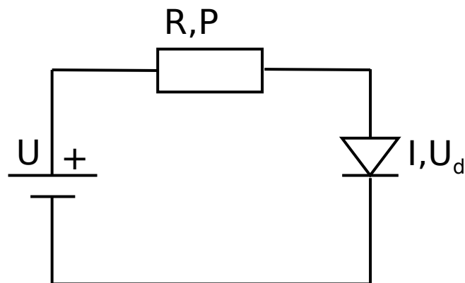
Рисунок 2.7 – Схема підключення діоду та резистору
