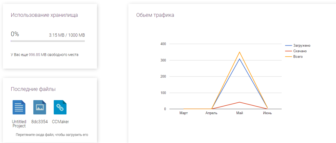
Рис.3.8. Сторінка статистики [ ]
