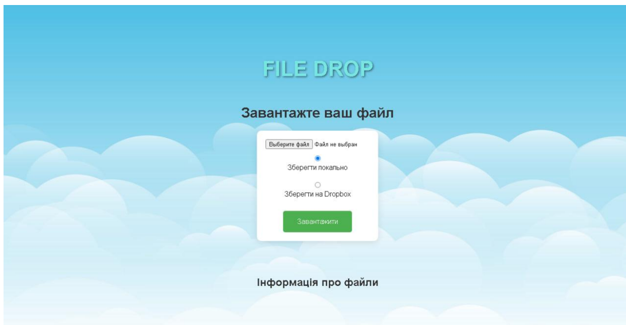
Рис.3.2 Головна сторінка [ ]
