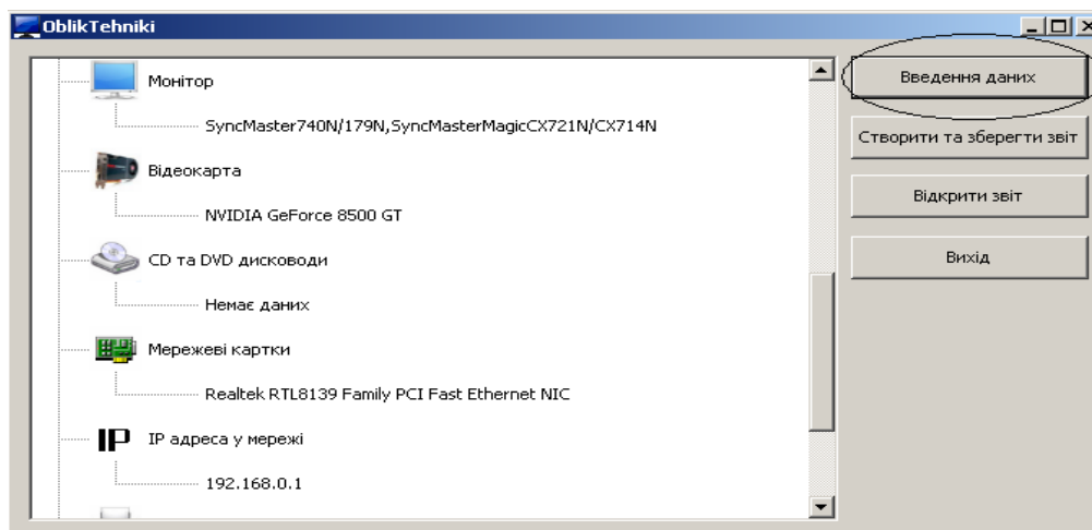
Рисунок 3.6. – Введення даних
