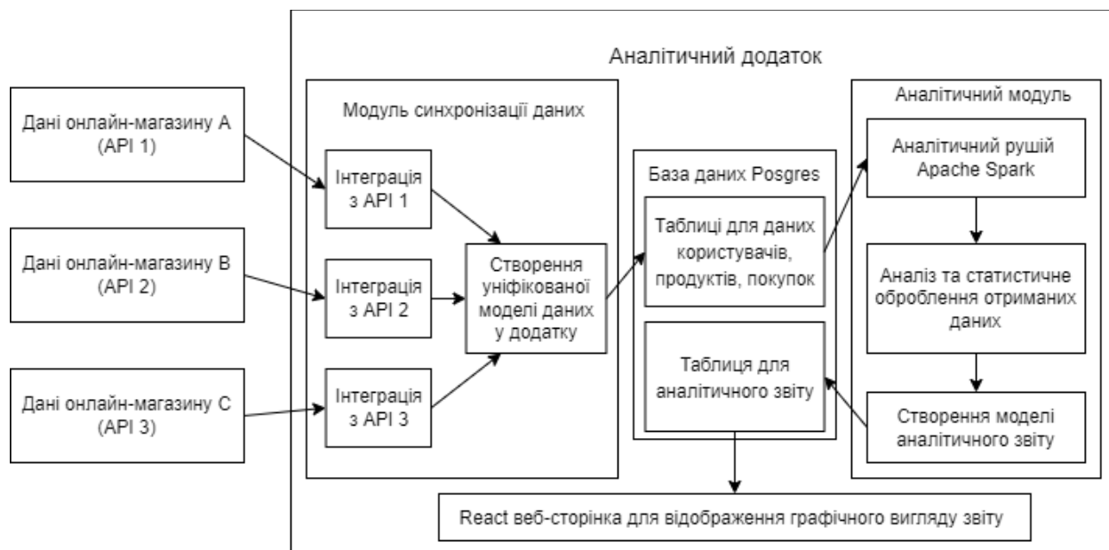
Рисунок 4.3 - Структурна схема додатку
