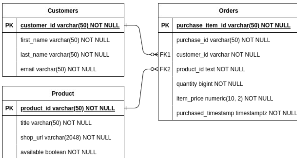
Рисунок 4.5 - Схема бази даних
