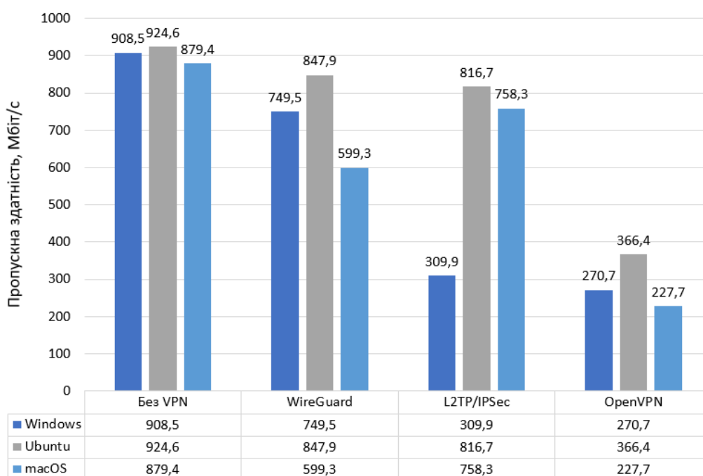
Рис. 3.1 – Тестування без деградацій мережі
