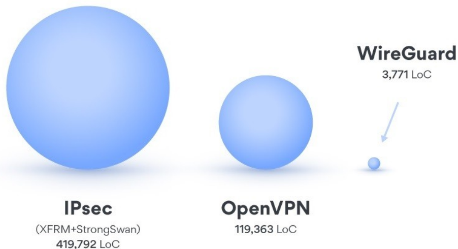
Рис. 2.1 – Порівняння кодової бази VPN-протоколів
