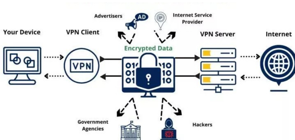
Рис. 1.6 – Ілюстрація VPN-шифрування
