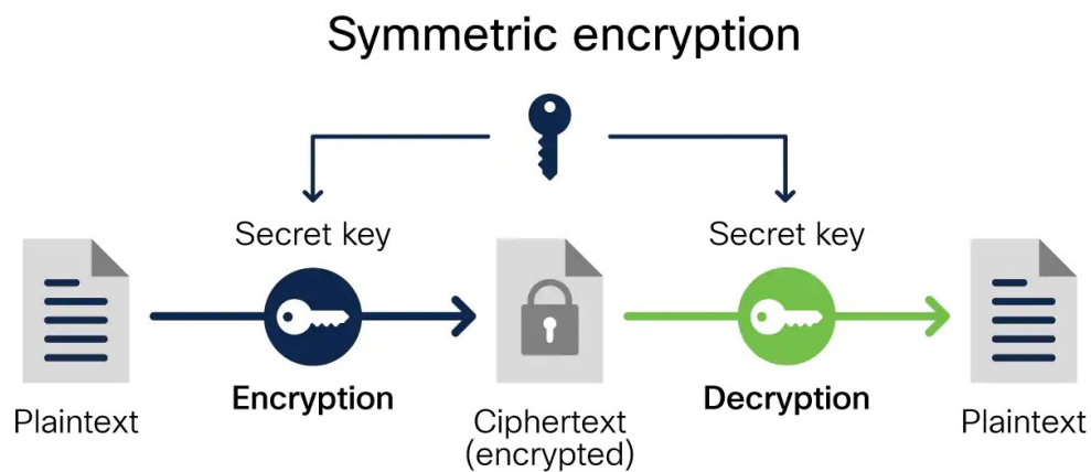
Рис. 1.7 – Симетричне шифрування
