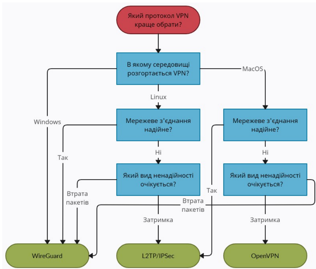
Рис. 3.4 – Дерево рішень
