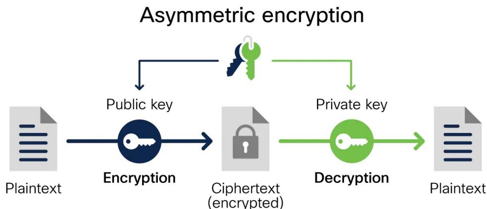
Рис. 1.8 – Асиметричне шифрування
