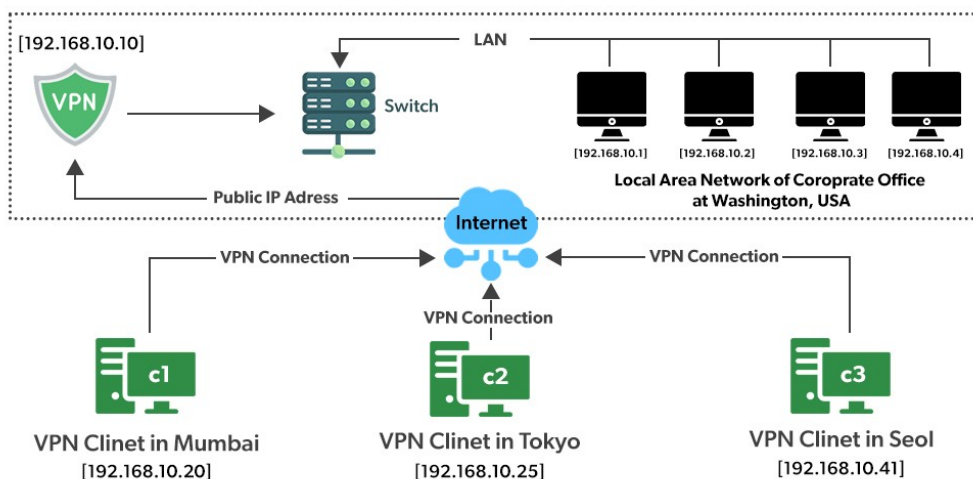
Рисунок 1.2 – Ілюстрація VPN
