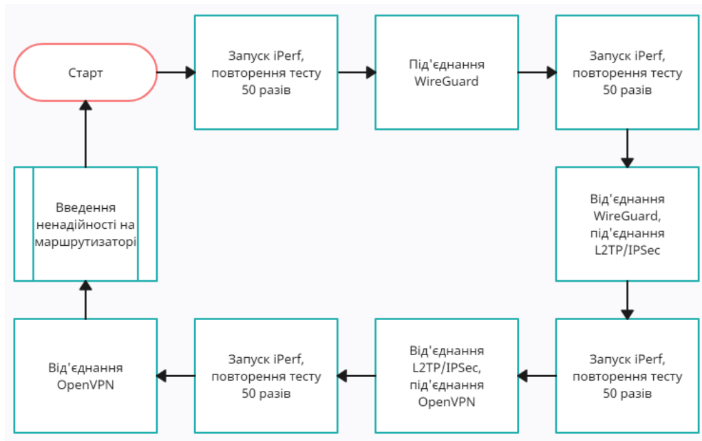
Рис. 2.5 – Блок-схема експерименту
