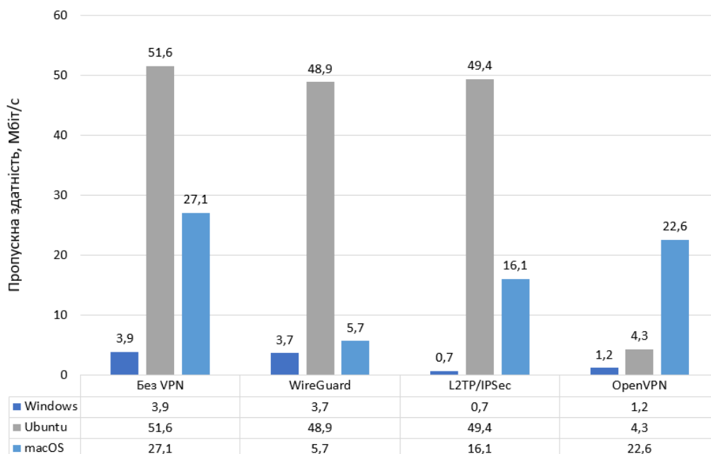
Рис. 3.2 – Тестування з першою ненадійністю
