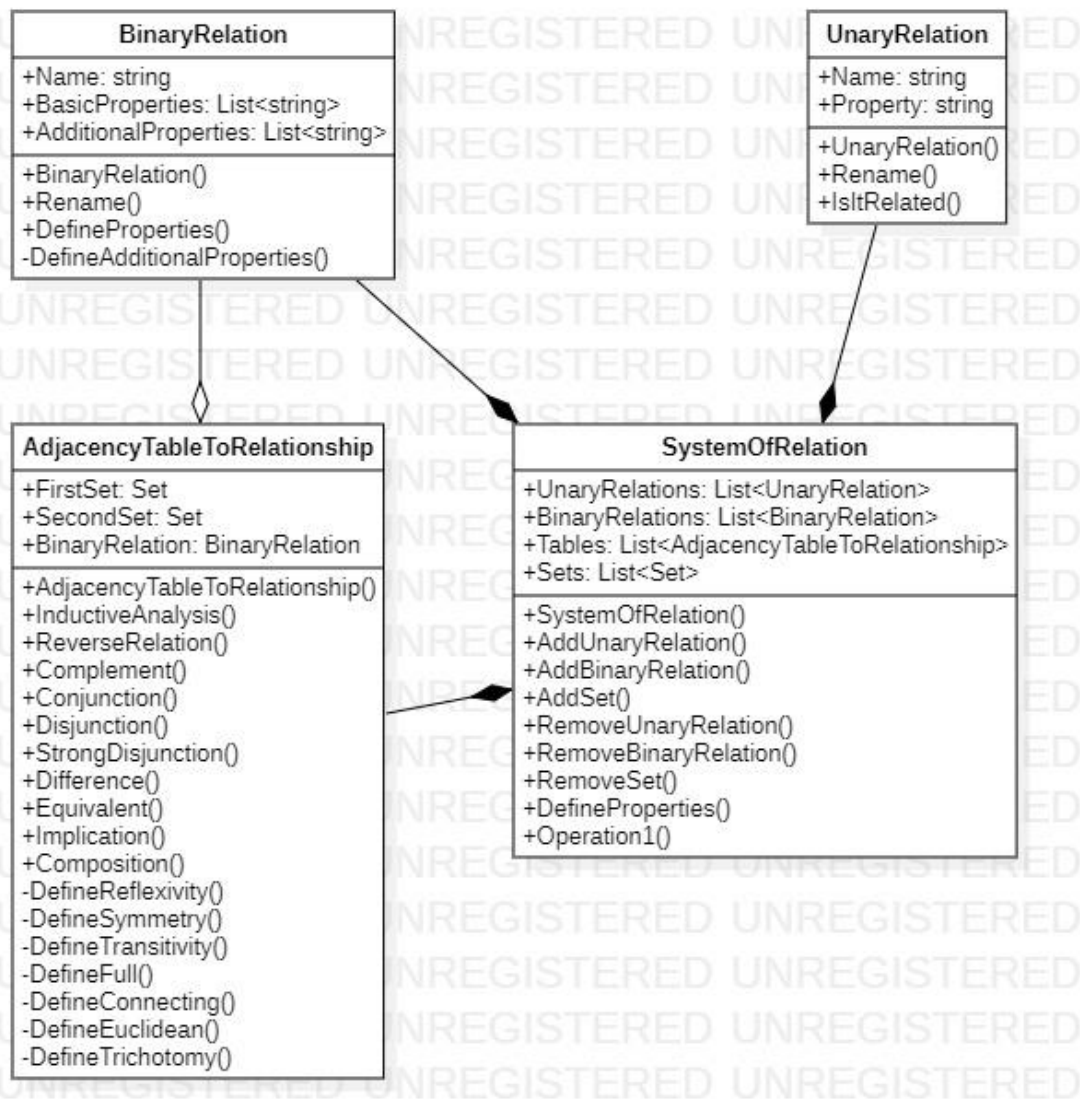
Рисунок 3.8 – Діаграма класів для представлення моделей теорії відношень
