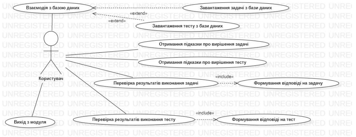
Рисунок 3.4 – Діаграма варіантів використання модуля для виконання задач та тестів
