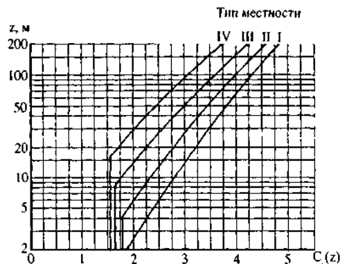
Рисунок 2.9 – Коефіцієнт висоти споруд C_h
