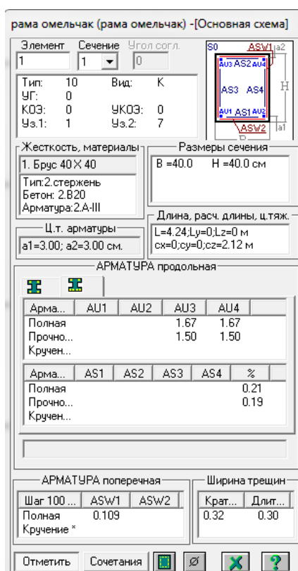
Рисунок 2.11. Результати підбору поздовжньої арматури:
