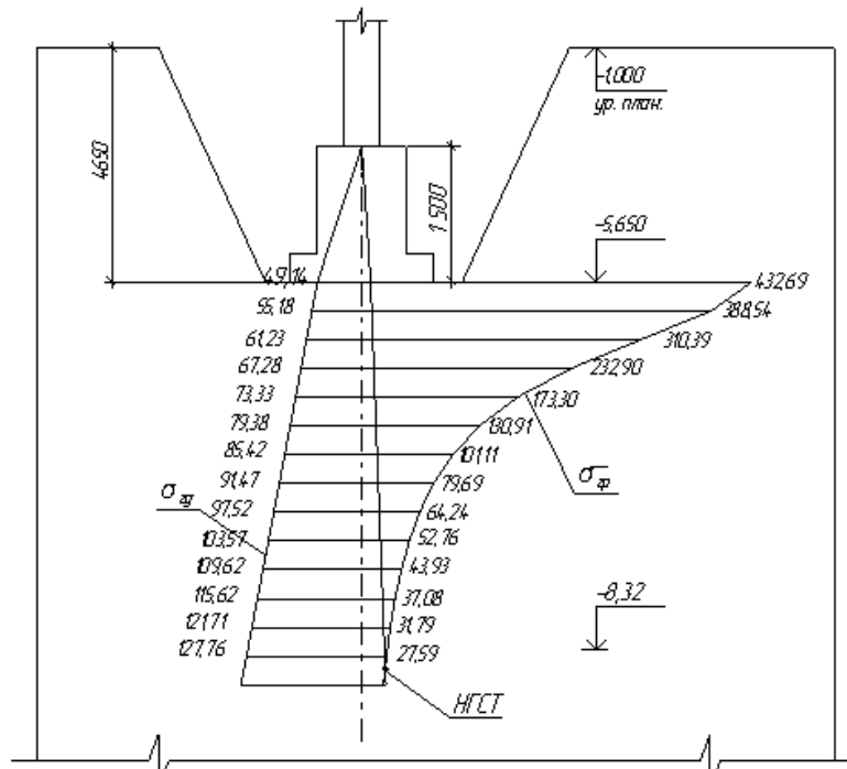
Рисунок 3.6 – Епюра природних і додаткових напруги окремого фундаменту
