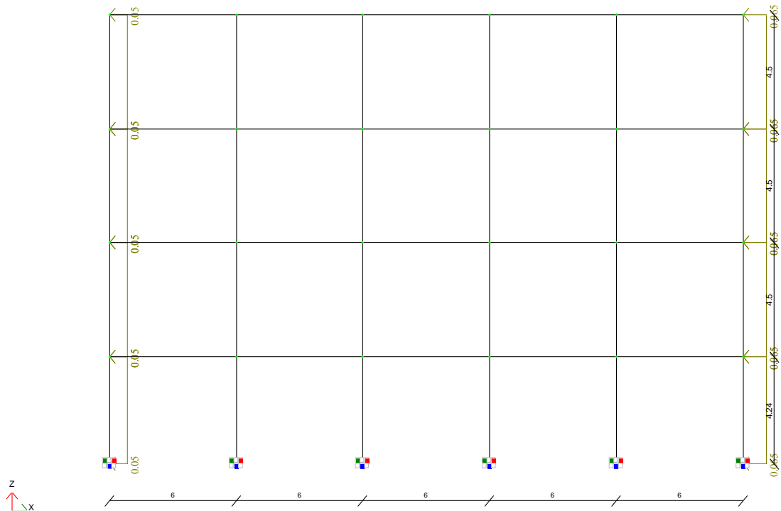
Рисунок 2.6. Схема завантаження №6 плоскої рами каркасу вітровим навантаженням.
