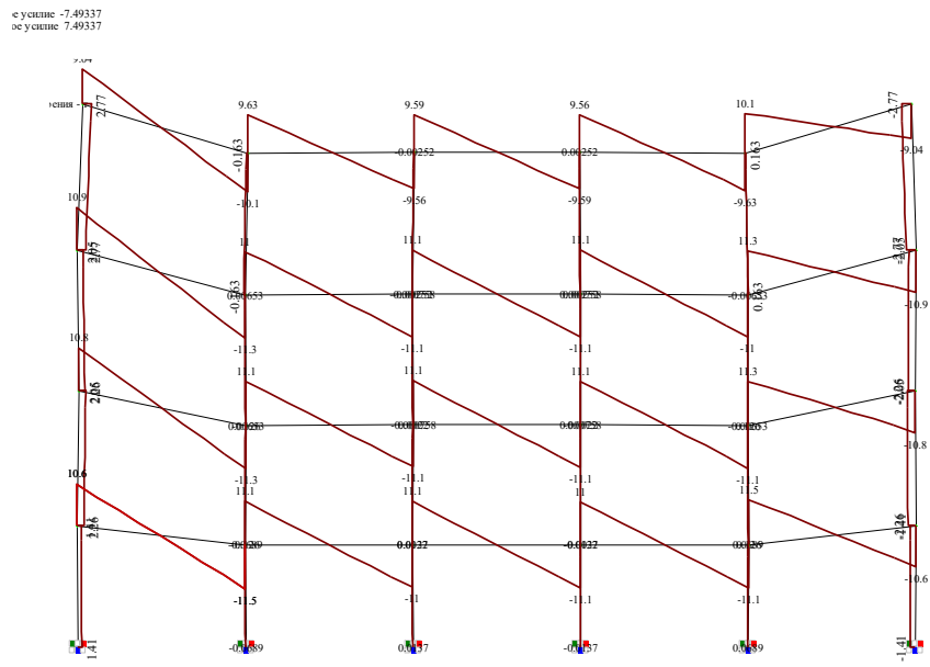
Рисунок 2.9 – Епюри поперечных сил
