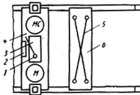
Рисунок 4.1 - Схема організації робочого місця при монтажі
