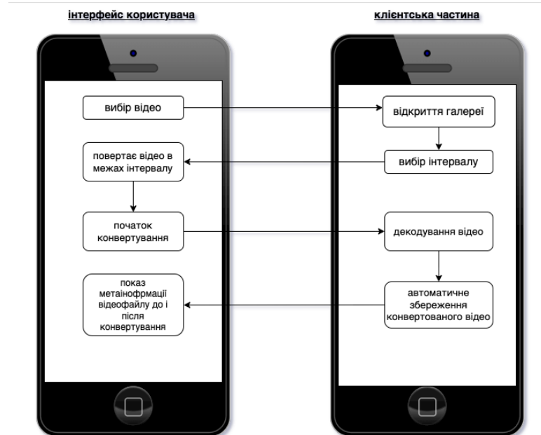
Рисунок 3.5 – Діаграма діяльності
