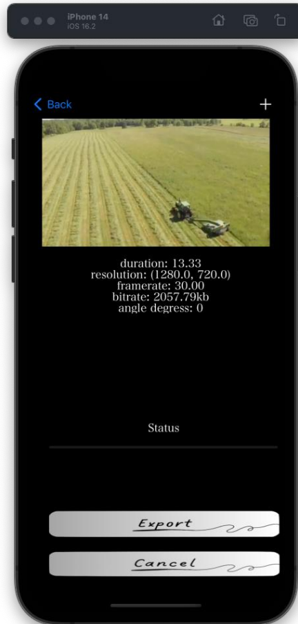
Рисунок 3.11 – Другий контролер
