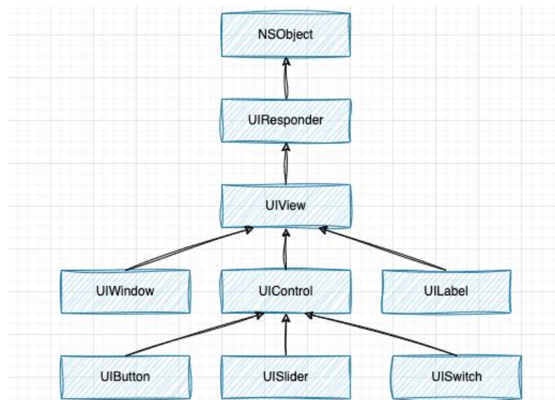
Рисунок 2.17 – UIKit Inheritance
