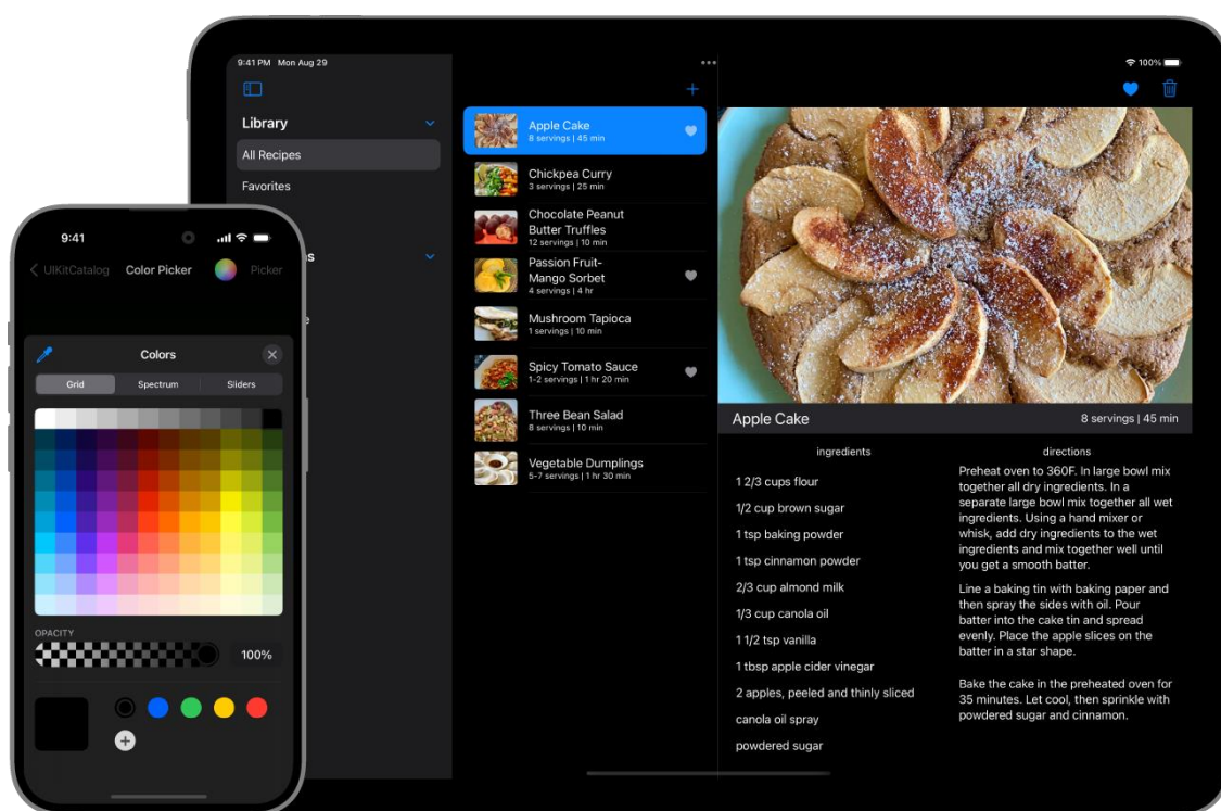
Рисунок 2.16 – Framework UIKit
