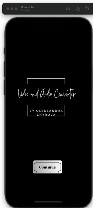
Рисунок 3.8 – Стартове вікно
