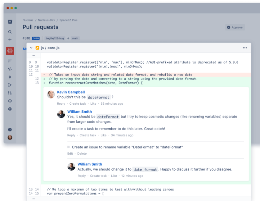
Рисунок 2.12 – програма Sourcetree
