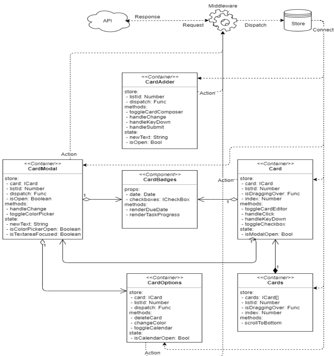
Рис. 2.17 – Діаграма компонентів Card модуля
