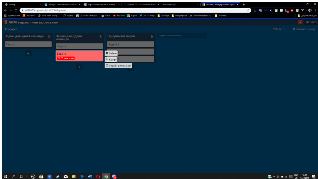
Рис. 3.24 – Параметри задачі
