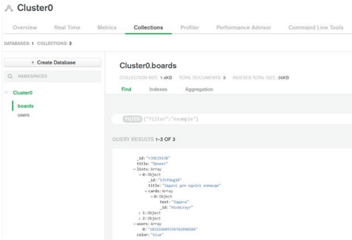
Рис 2.12 – Список дошок
