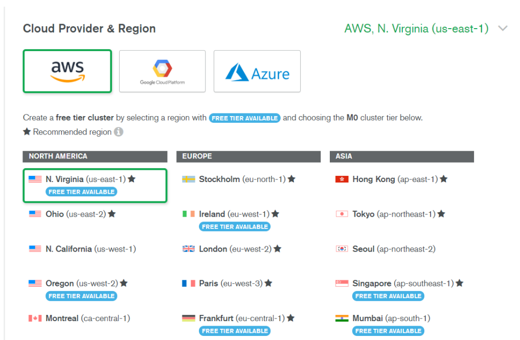
Рис 2.2 – Вибір регіону
