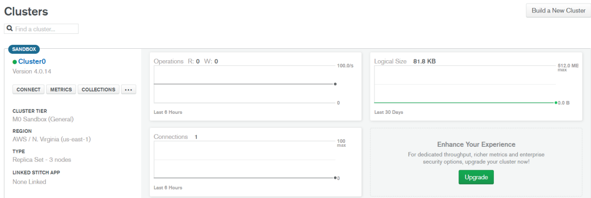
Рис 2.5 – Властивості кластеру
