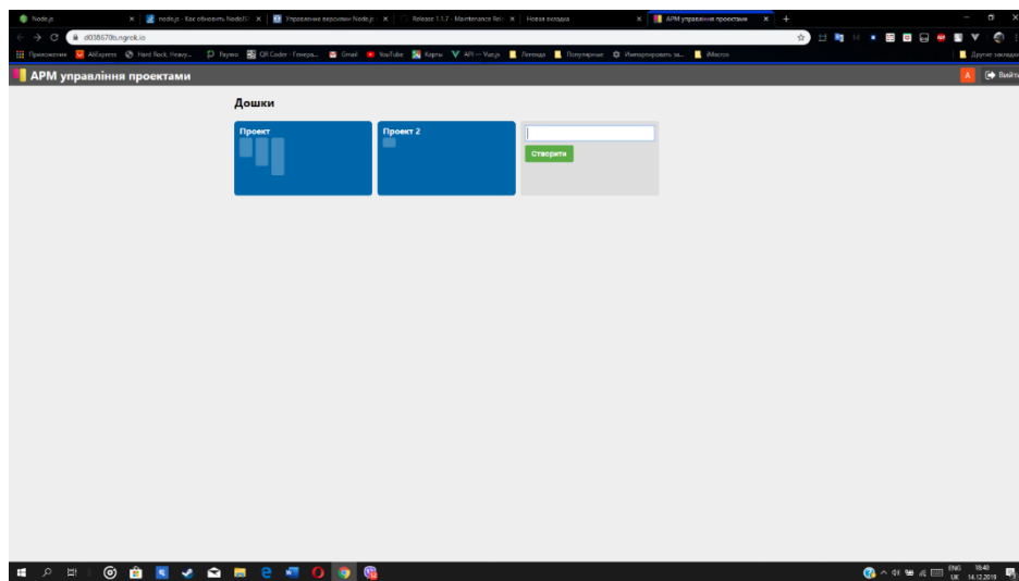
Рис. 3.27 – Додавання дошки
