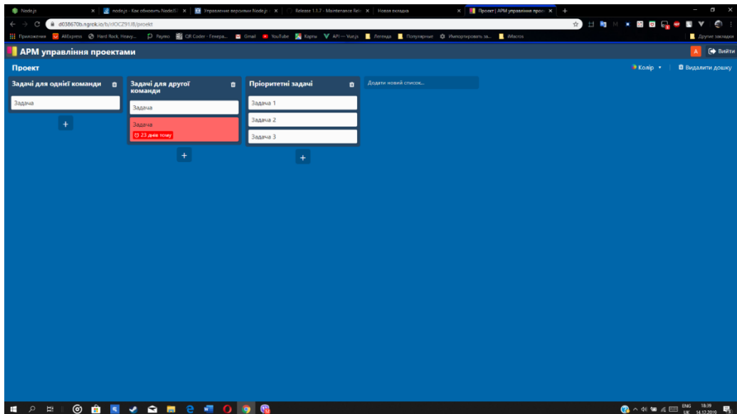
Рис. 3.22 – Задачі проекту
