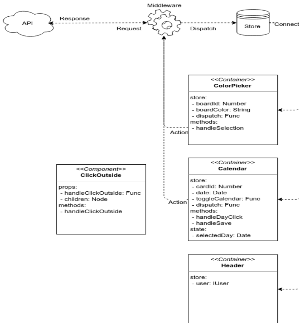
Рис. 2.18 – Діаграма компонентів Shared модуля
