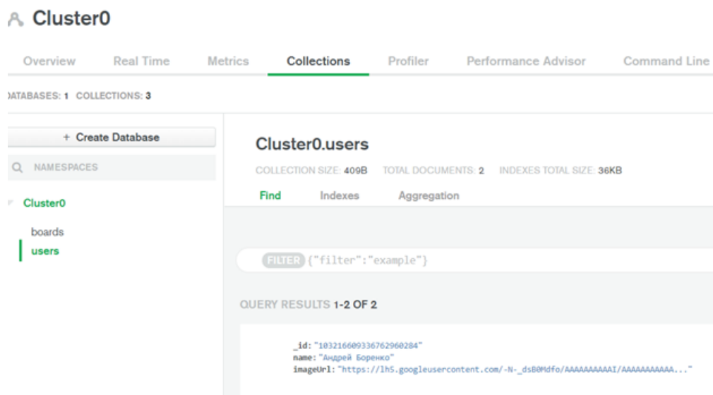
Рис 2.10 – Список користувачів
