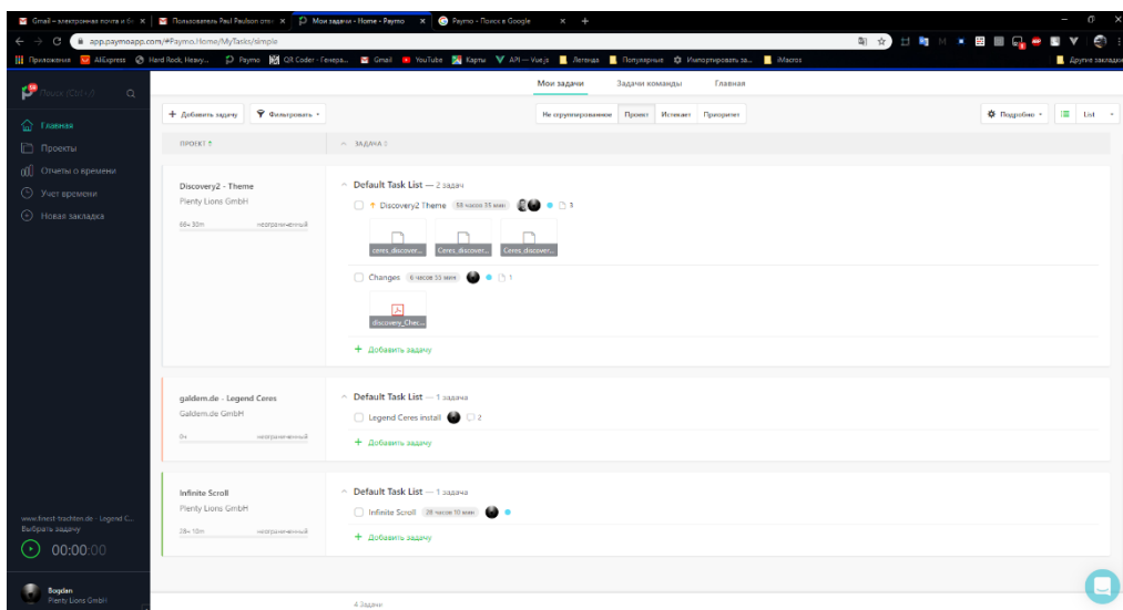
Рис. 1.3 – Інтерфейс Раутоарр
